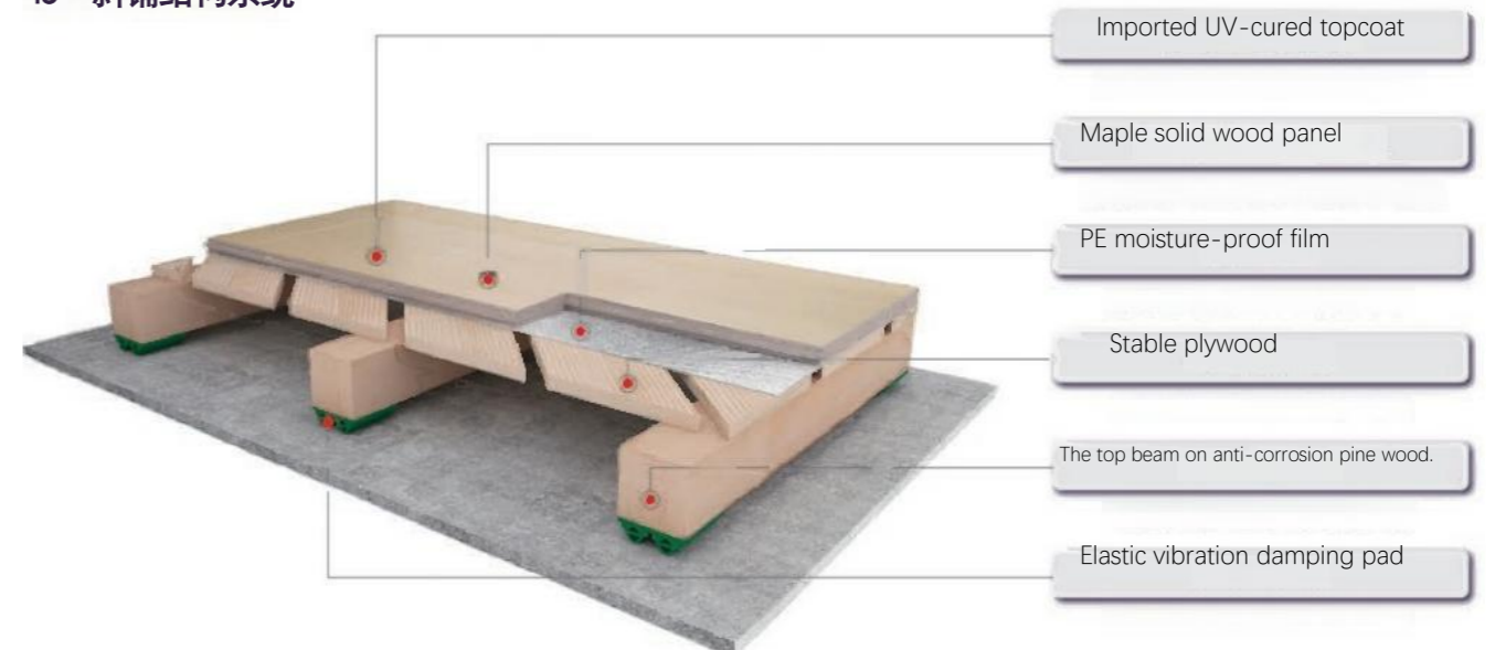
45° 斜铺结构系统
